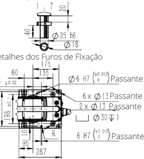
Detalhes dos Furos de Montagem da Base
